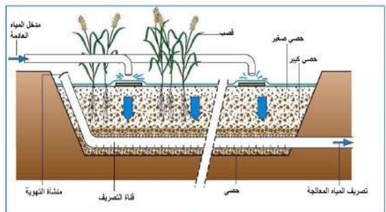
Principe de fonctionnement des filtres plantés de roseaux (Source : Agence de l'Eau - méditerranée - Corse)
